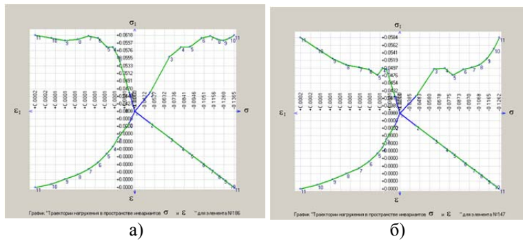
Рис. 3. Графики траекторий нагружения для верхнего КЭ нижнего слоя асфальтобетона в сечении №1: а) схема 1; б) схема 2
